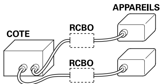
Raccordement avec deux RCBO
