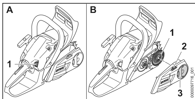
Kraftstoffhandpumpe (A)
